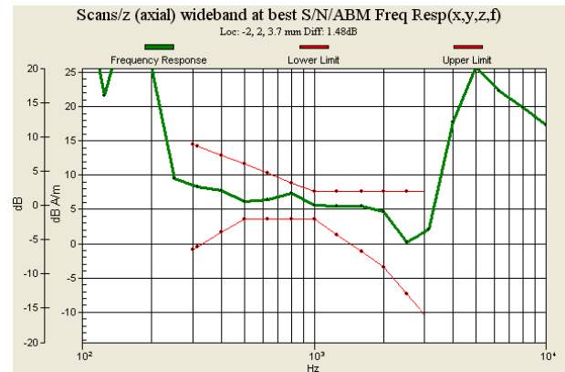
Fig. 9.2 GSM850 Ch189
