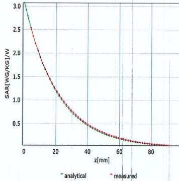
f=750 MHz,WGLS R9(H_convF)
