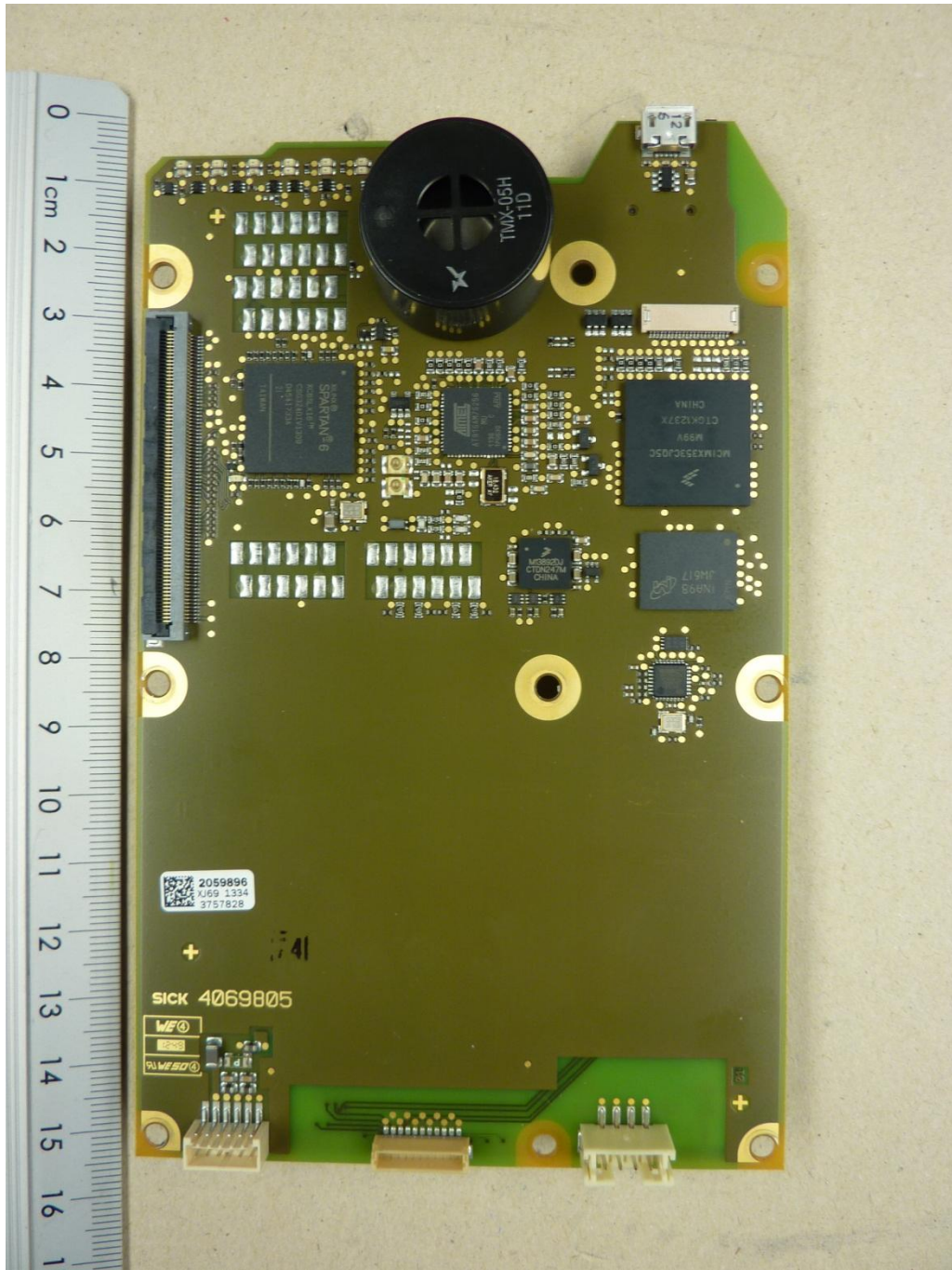
135012_7.JPG: RFU630 PCB 1, top view
