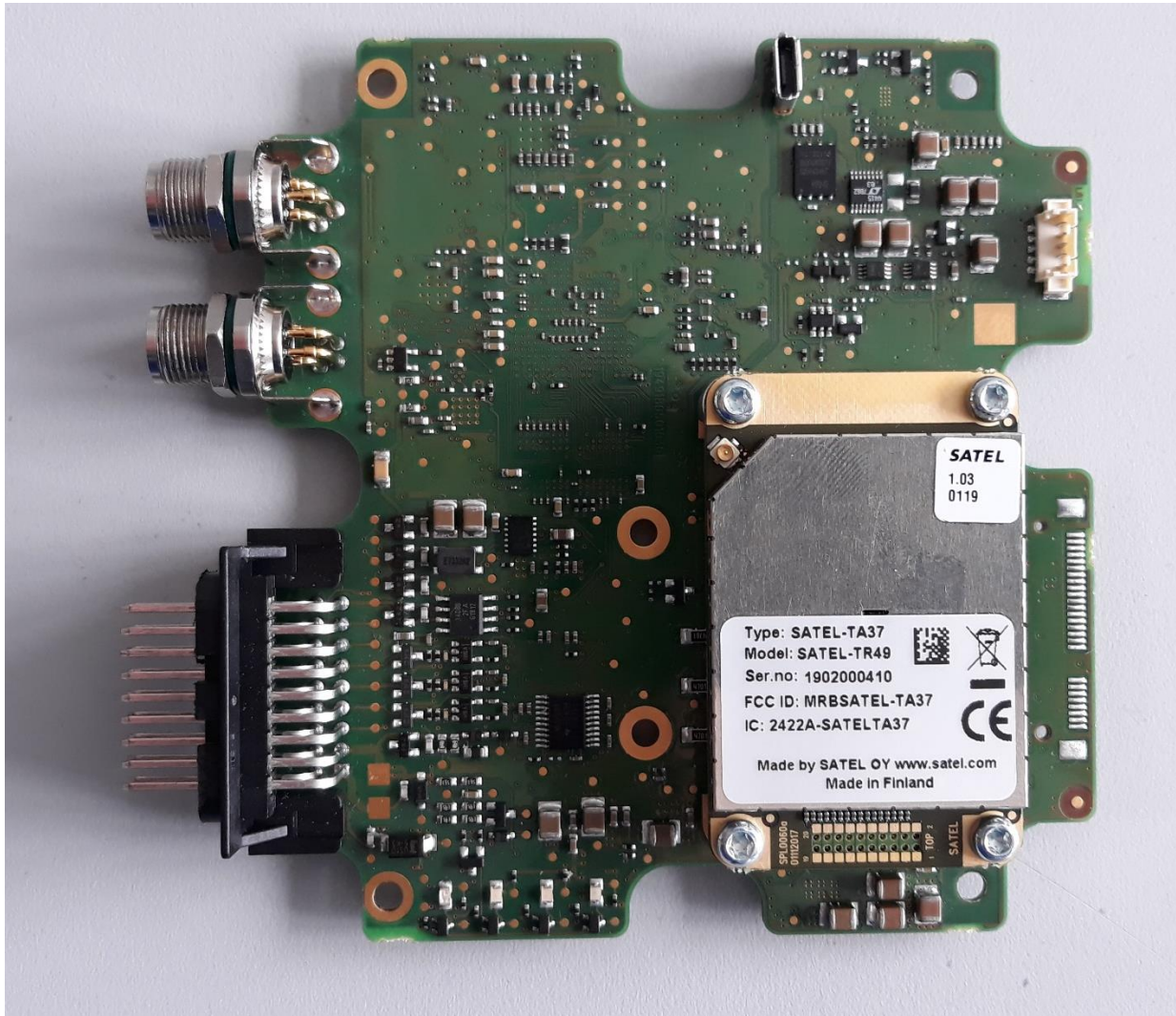
Satel Oy type SATEL-TA37
