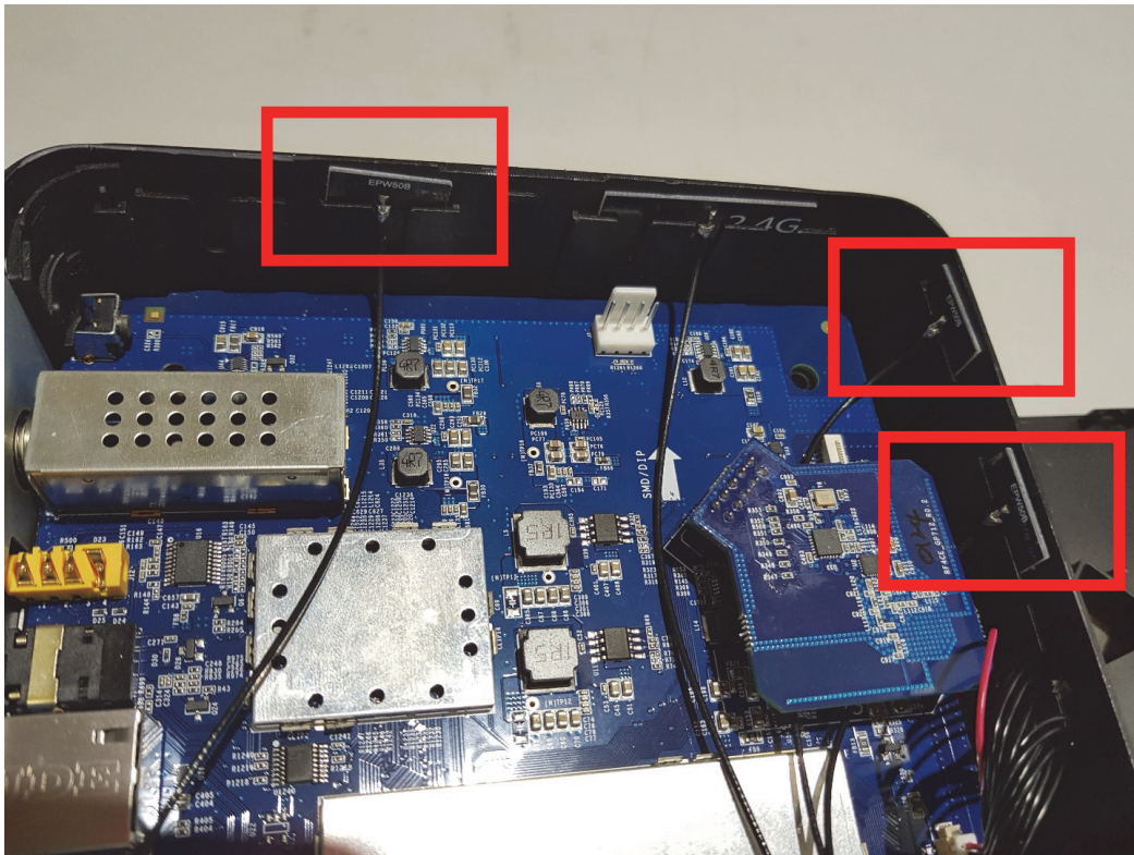
WLAN 5GHz_Antenna 0/1/2
