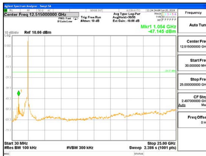
802.11n_HT20_ANT2
