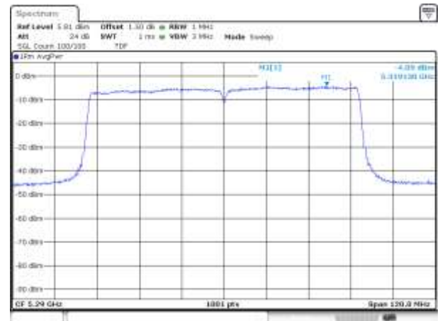
UNII-2A / 802.11ac VHT80 / 5 290 MHz
