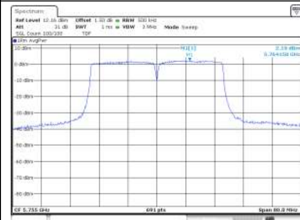
UNII-3 / 802.11ac VHT40 / 5 755 MHz
