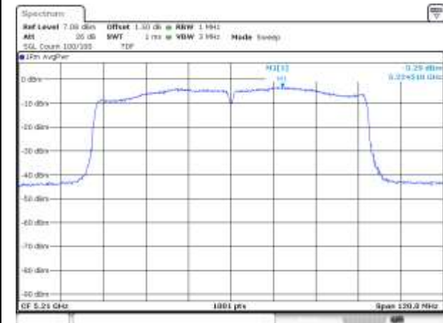
UNII-1 / 802.11ac VHT80 / 5 210 MHz
