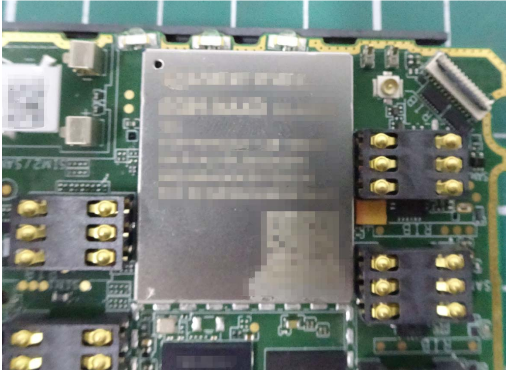
WWAN Module
