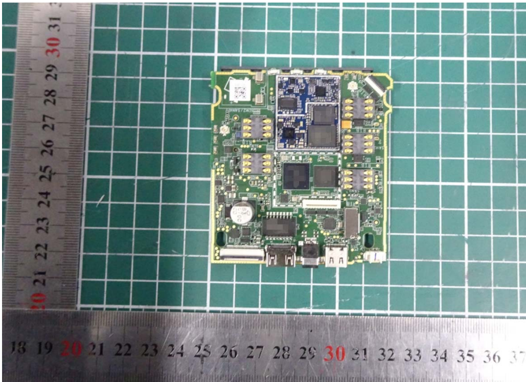
WWAN Module
