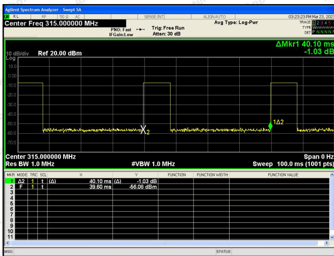
315MHz(FSK)-T period
