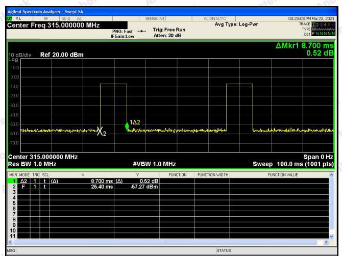
315MHz(FSK)-T on1
