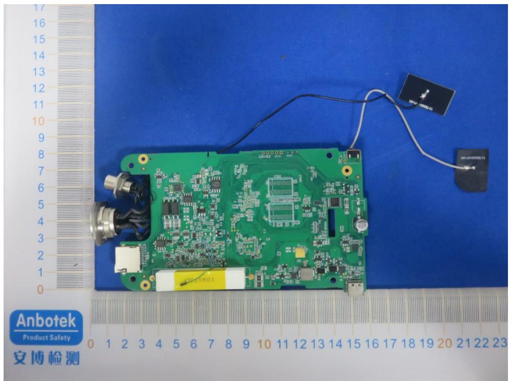
BT ANT
