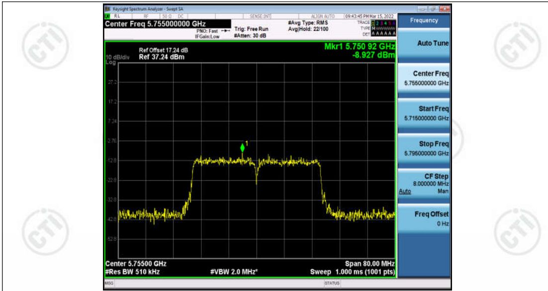
11N40MIMO_Ant1_5755
