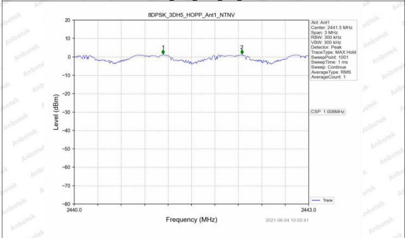
8DPSK_3DH5_HOPP_Ant1_NTNV
