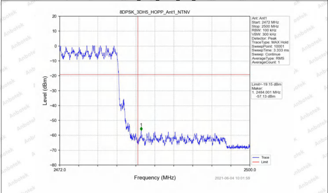
8DPSK_3DH5_HOPP_Ant1_NTNV
