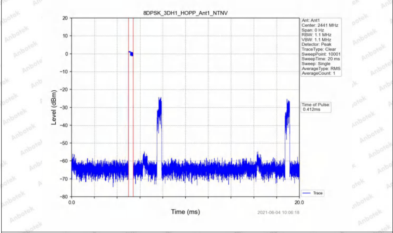
8DPSK_3DH1_HOPP_Ant1_NTNV
