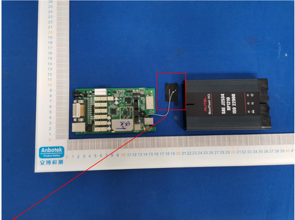
BT ANT
