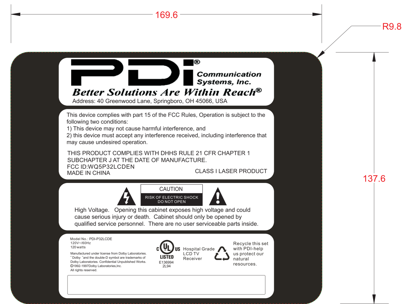
后壳表牌 零件号:LT-93201-H02
