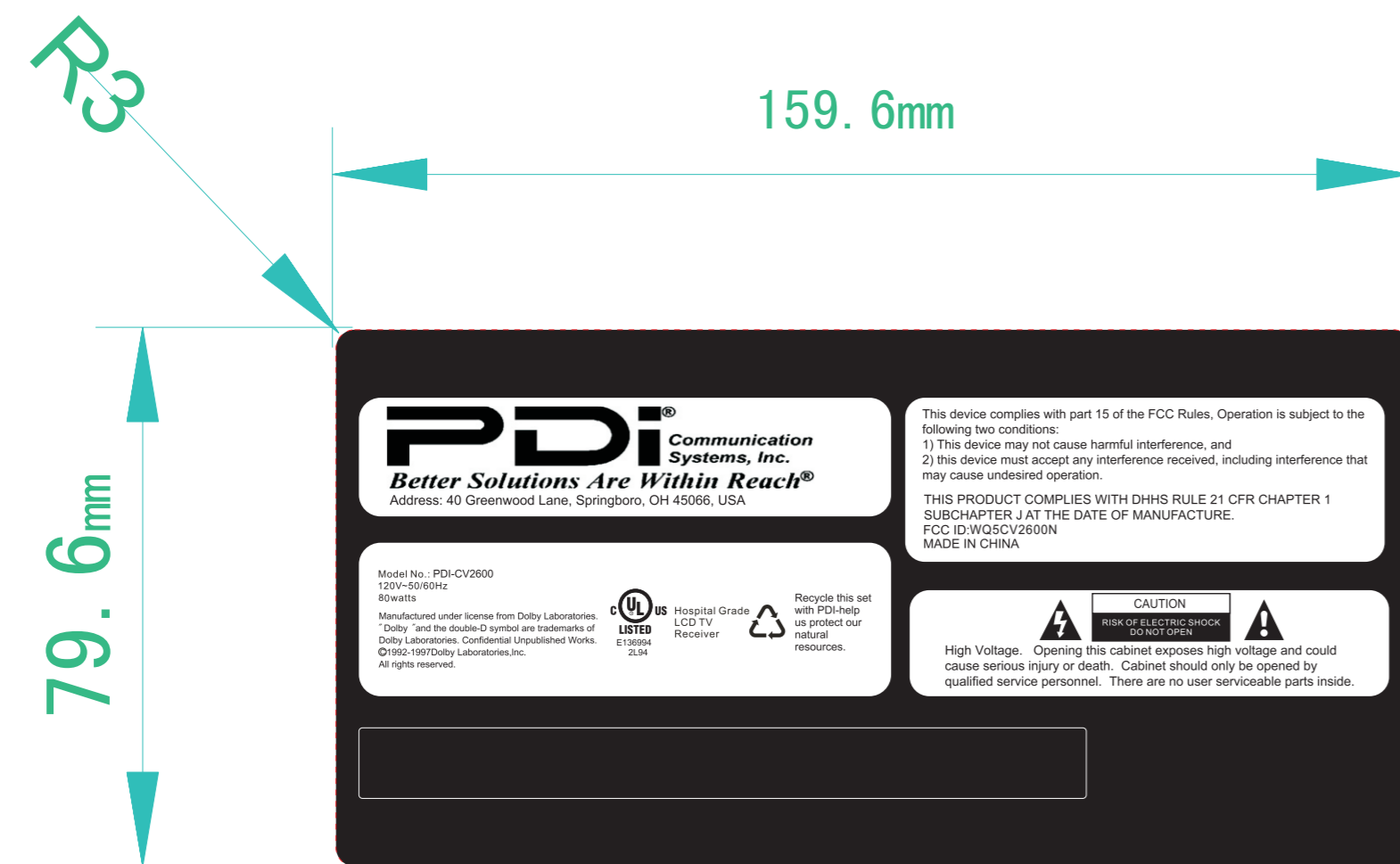
后壳表牌
