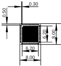
Abbildung 1: EINTLEG Dimensions
