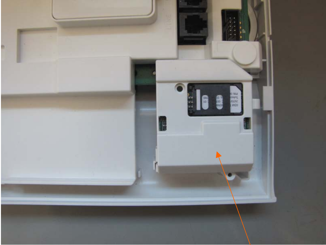
GSM modem
