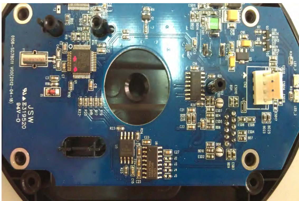
< PCB6-F >
