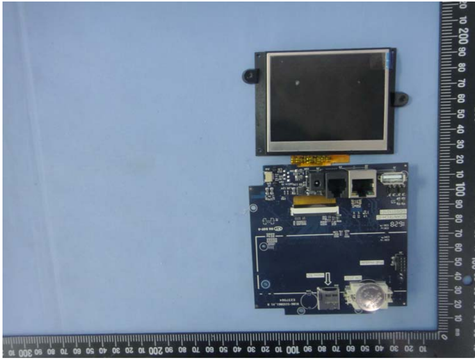
EUT Photo 26 )
