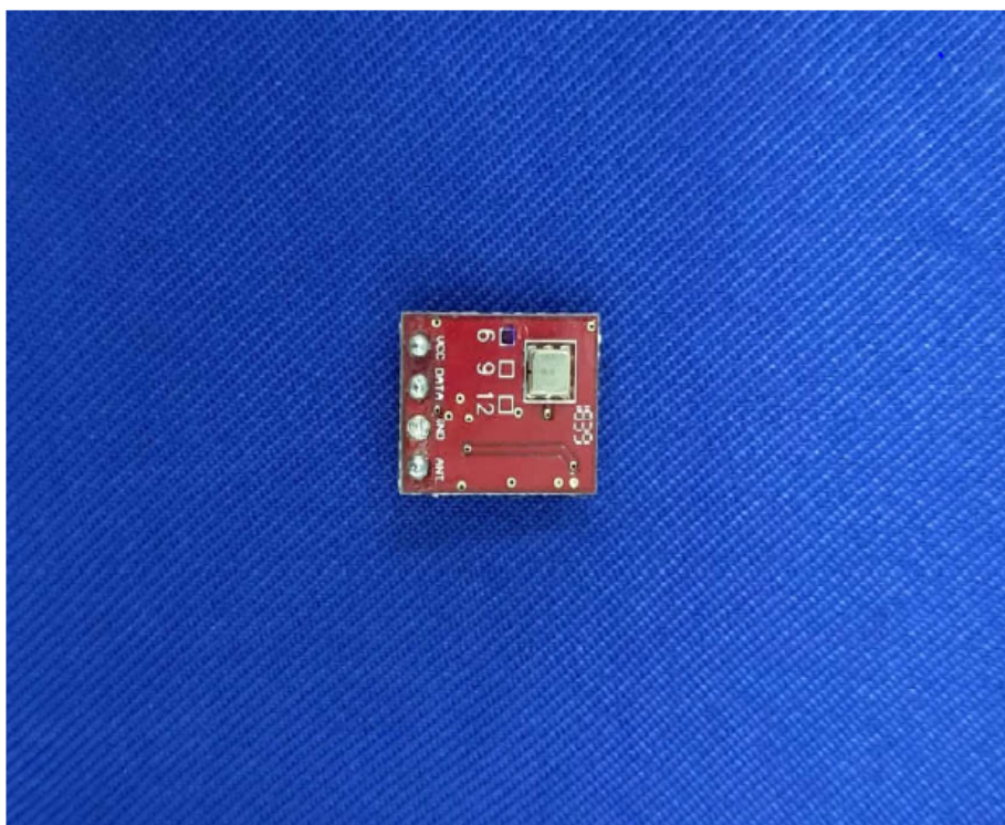
RF Module
