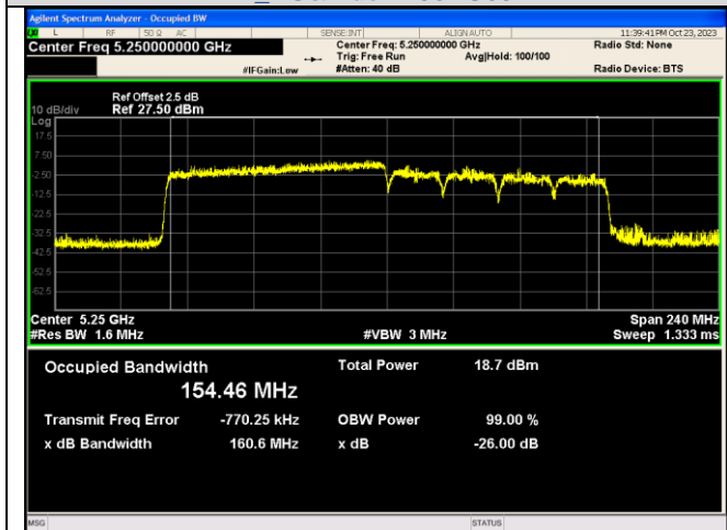
IEEE 802.11ax_Channel 50_160MHz_Antenna 2_RU&Index 996RU67
