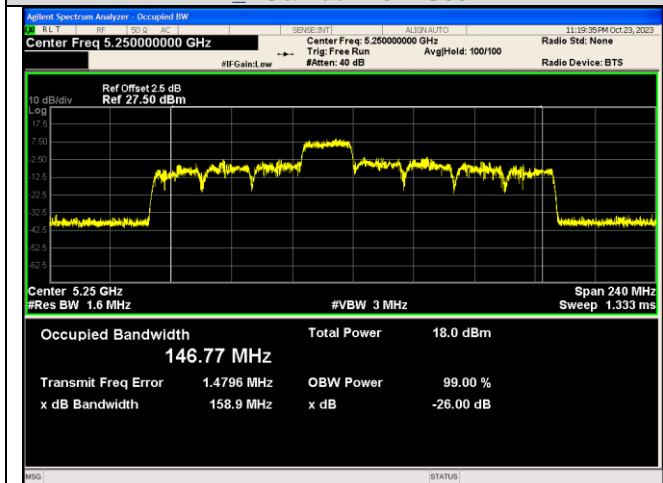
IEEE 802.11ax_Channel 50_160MHz_Antenna 2_RU&Index 242RU64
