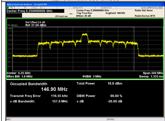
IEEE 802.11ax_Channel 50_160MHz_Antenna 2_RU&Index 106RU60
