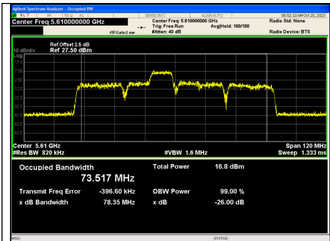
IEEE 802.11ax_Channel 122_80MHz_Antenna 2_RU&Index 106RU56
