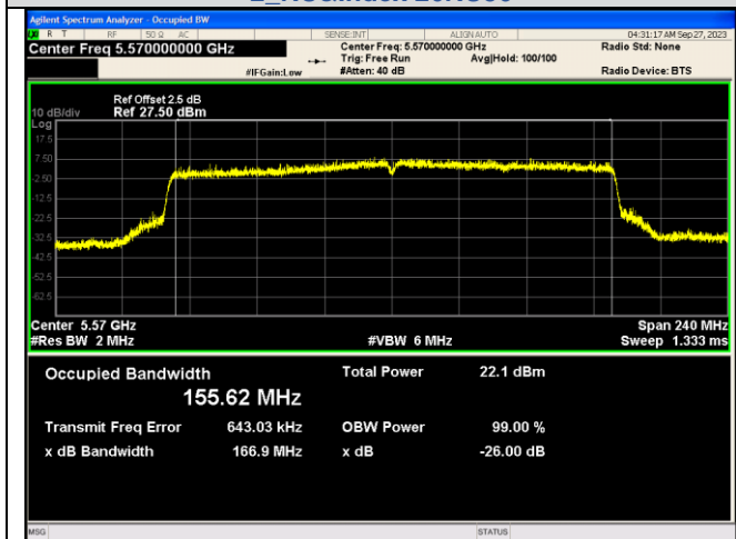
IEEE 802.11ax_Channel 114_160MHz_Antenna 2_RU&Index 996*2RU68
