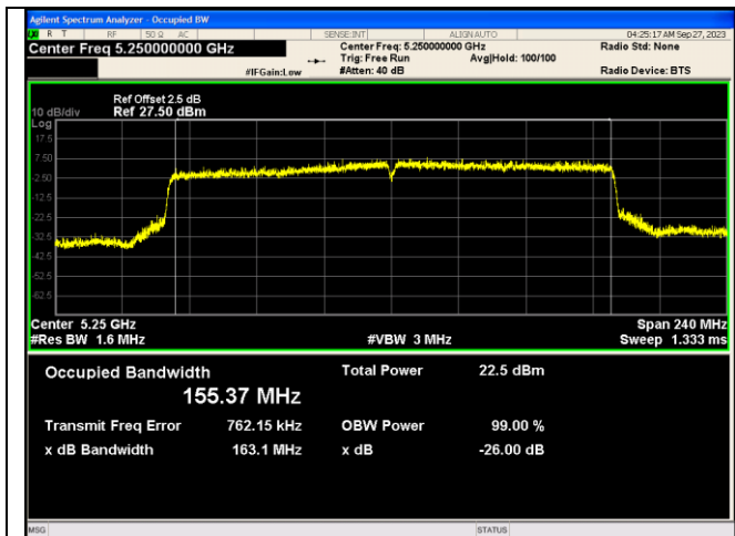
IEEE 802.11ax_Channel 50_160MHz_Antenna 2_RU&Index 996*2RU68
