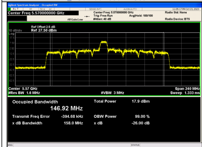
IEEE 802.11ax_Channel 114_160MHz_Antenna 2_RU&Index 106RU60
