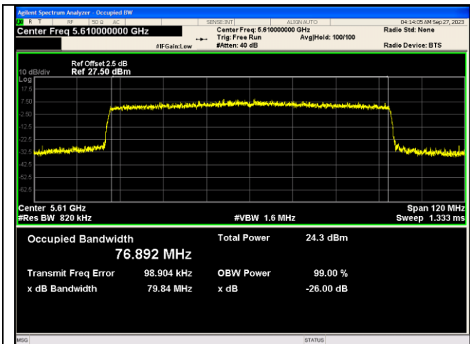
IEEE 802.11ax Channel 122 80MHz Antenna 2 RU&Index 996RU67
