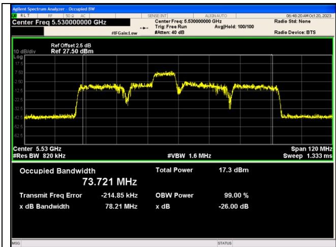
IEEE 802.11ax_Channel 106_80MHz_Antenna 2_RU&Index 106RU56
