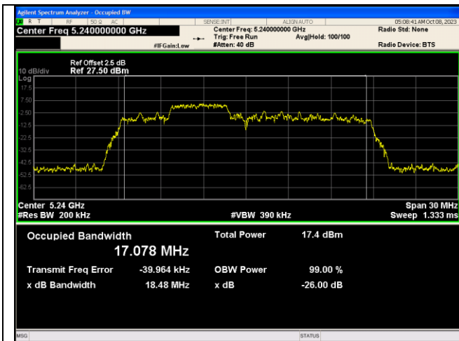
IEEE 802.11ax_Channel 48_20MHz_Antenna 0_RU&Index 52RU38
