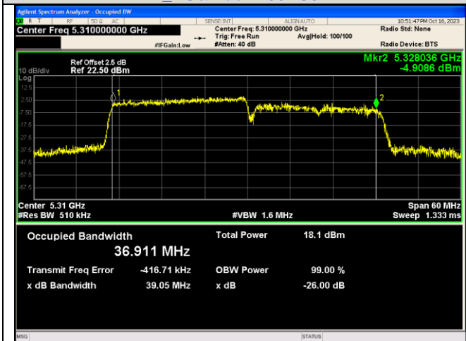
IEEE 802.11ax_Channel 62_40MHz_Antenna 2_RU&Index 242RU61
