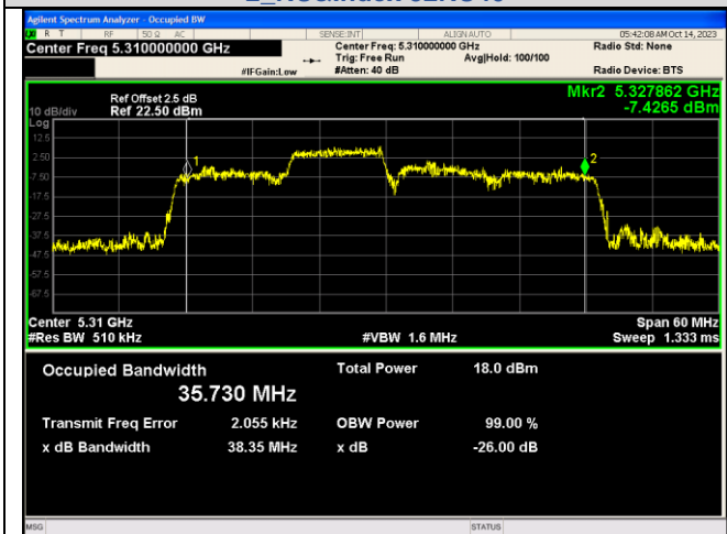
IEEE 802.11ax_Channel 62_40MHz_Antenna 2_RU&Index 106RU54
