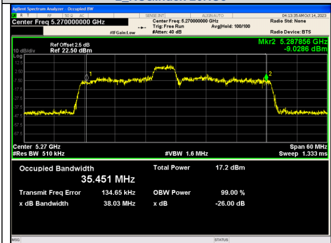
IEEE 802.11ax_Channel 54_40MHz_Antenna 2 RU&Index 52RU40
