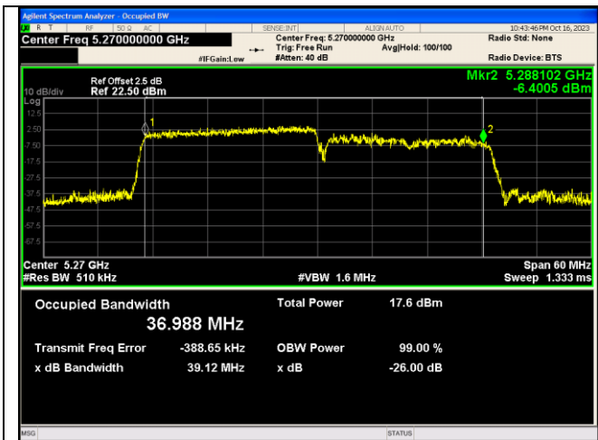
IEEE 802.11ax_Channel 54_40MHz_Antenna 2_RU&Index 242RU61
