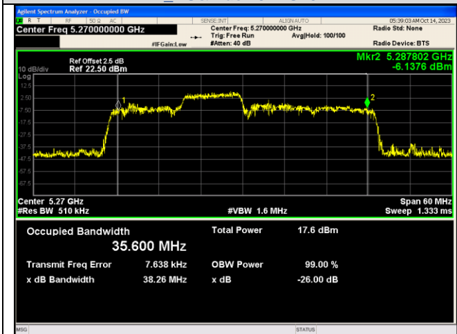
IEEE 802.11ax_Channel 54_40MHz_Antenna 2 RU&Index 106RU54
