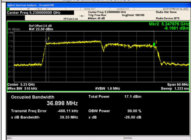
IEEE 802.11ax_Channel 46_40MHz_Antenna 2_RU&Index 242RU61
