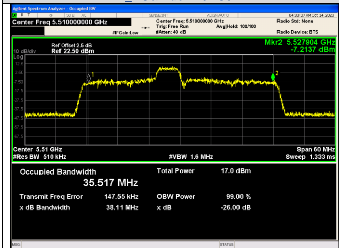
IEEE 802.11ax_Channel 102_40MHz_Antenna 2_RU&Index 52RU40
