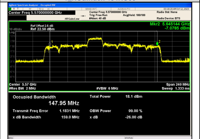
IEEE 802.11ax_Channel 114_160MHz_Antenna 1_RU&Index 242RU64
