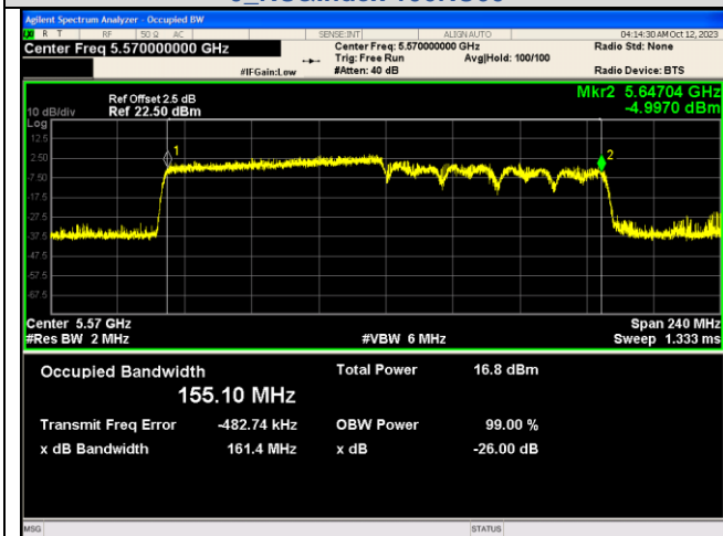
IEEE 802.11ax_Channel 114_160MHz_Antenna 0_RU&Index 996RU67
