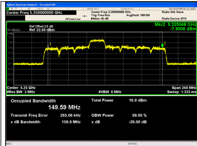
IEEE 802.11ax_Channel 50_160MHz_Antenna 0_RU&Index 242RU64
