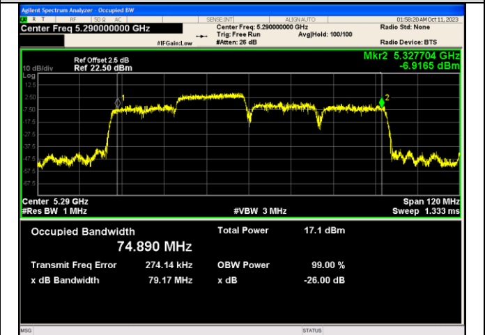
IEEE 802.11ax_Channel 58_80MHz_Antenna 1_RU&Index 242RU62
