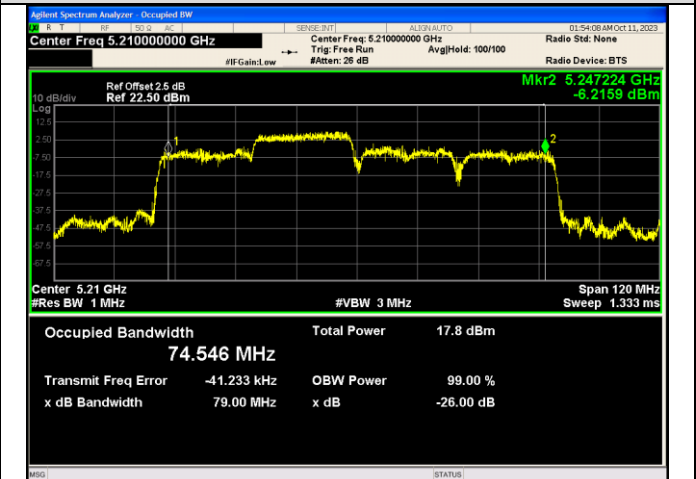
IEEE 802.11ax_Channel 42_80MHz_Antenna 1_RU&Index 242RU62
