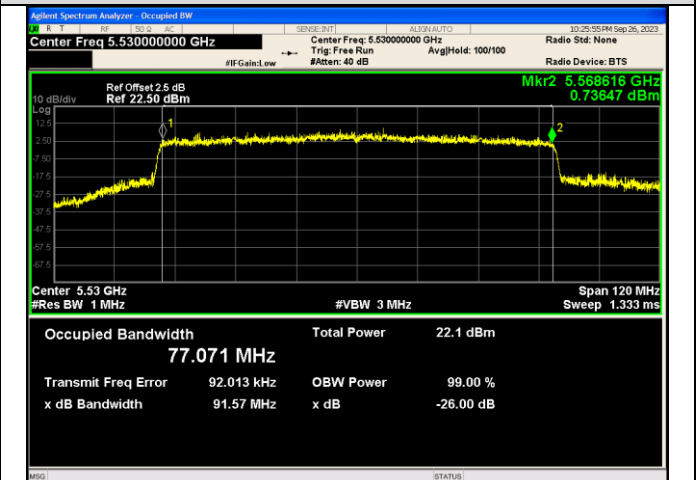
IEEE 802.11ax_Channel 106_80MHz_Antenna 1_RU&Index 996RU67
