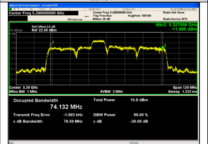
IEEE 802.11ax_Channel 58_80MHz_Antenna 1_RU&Index 106RU56
