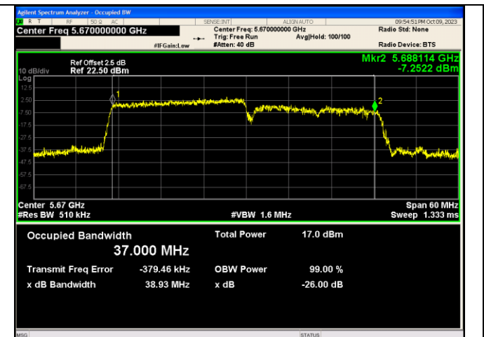
IEEE 802.11ax_Channel 134_40MHz_Antenna 1_RU&Index 242RU61
