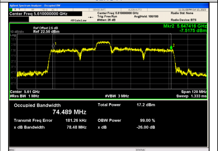
IEEE 802.11ax_Channel 122_80MHz_Antenna 1_RU&Index 106RU56
