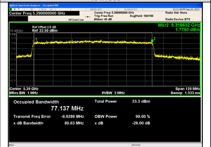
IEEE 802.11ax_Channel 58_80MHz_Antenna 1_RU&Index 996RU67
