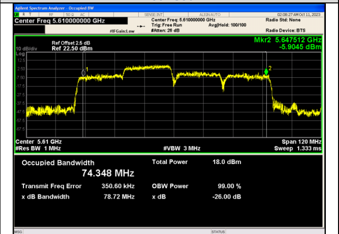
IEEE 802.11ax_Channel 122_80MHz_Antenna 1_RU&Index 242RU62
