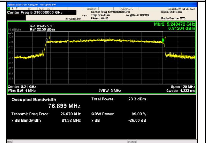
IEEE 802.11ax_Channel 42_80MHz_Antenna 1_RU&Index 996RU67
