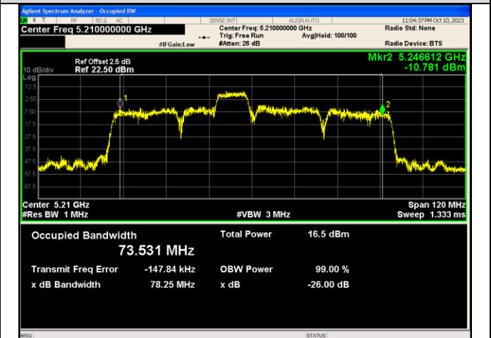
IEEE 802.11ax_Channel 42_80MHz_Antenna 1_RU&Index 106RU56
