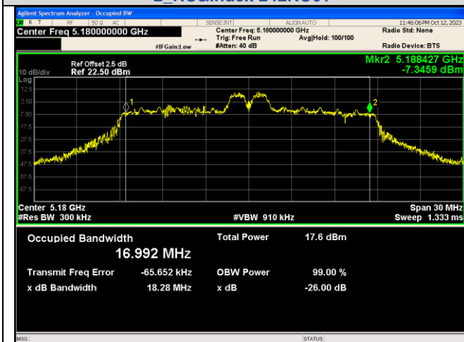
IEEE 802.11ac_Channel 36_20MHz_Antenna 2_RU&Index 26RU4
