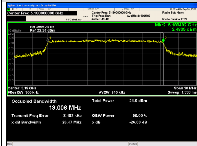
IEEE 802.11ac_Channel 36_20MHz_Antenna 2_RU&Index 242RU61
