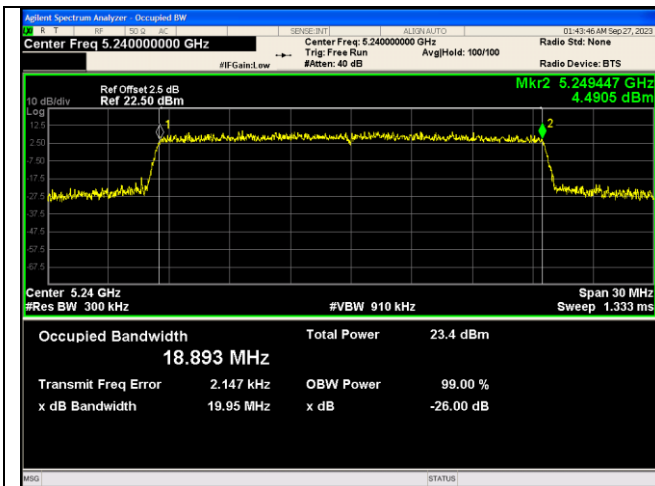
IEEE 802.11ax_Channel 48_20MHz_Antenna 2_RU&Index 242RU61
