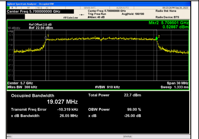
IEEE 802.11ax_Channel 140_20MHz_Antenna 1_RU&Index 242RU61
