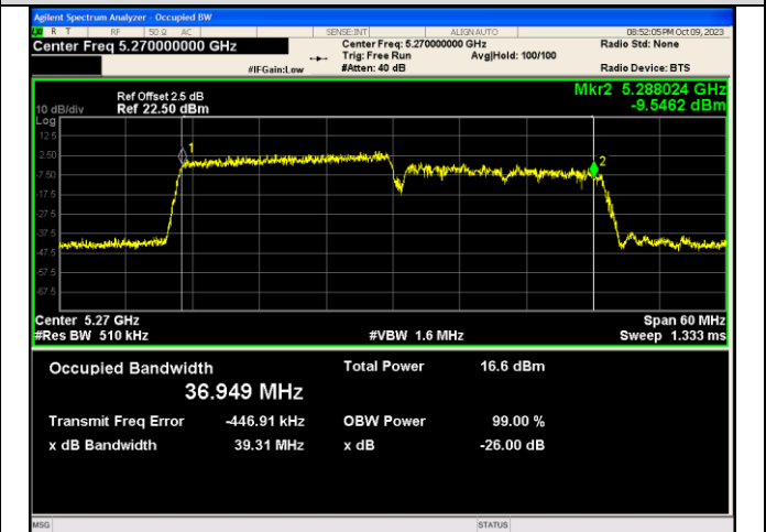
IEEE 802.11ax_Channel 54_40MHz_Antenna 1_RU&Index 242RU61
