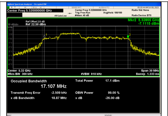
IEEE 802.11ax_Channel 64_20MHz_Antenna 1_RU&Index 52RU38
