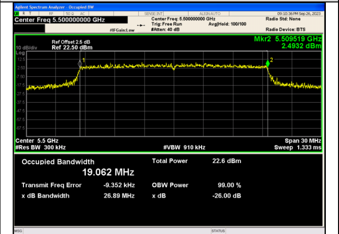
IEEE 802.11ax_Channel 100_20MHz_Antenna 1_RU&Index 242RU61
