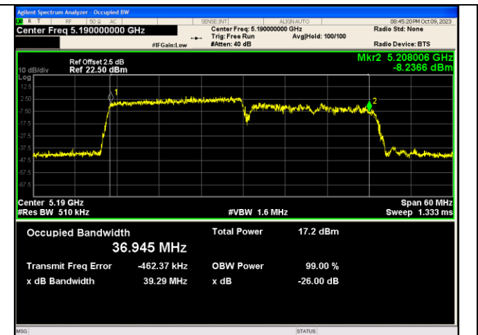
IEEE 802.11ax_Channel 38_40MHz_Antenna 1_RU&Index 242RU61
