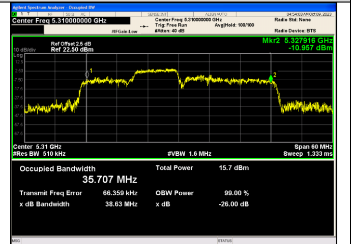
IEEE 802.11ax_Channel 62_40MHz_Antenna 1_RU&Index 106RU54
