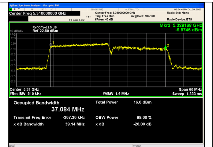
IEEE 802.11ax_Channel 62_40MHz_Antenna 1_RU&Index 242RU61
