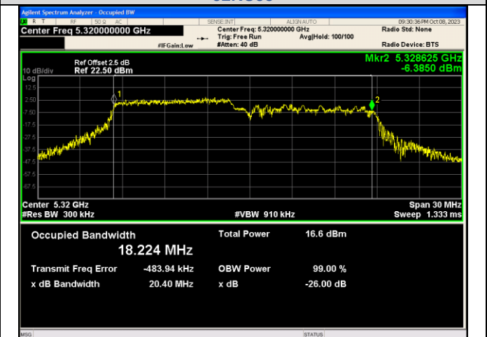
IEEE 802.11ax_Channel 64_20MHz_Antenna 1_RU&Index 106RU53
