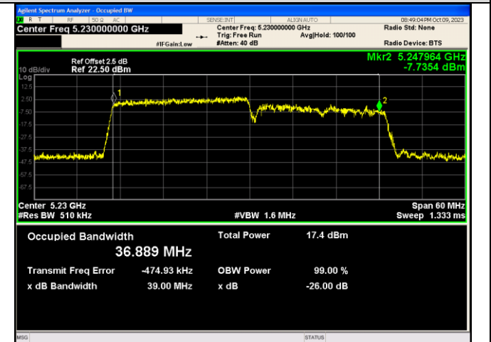
IEEE 802.11ax_Channel 46_40MHz_Antenna 1_RU&Index 242RU61
