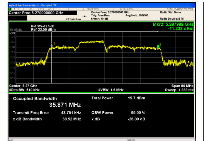
IEEE 802.11ax_Channel 54_40MHz_Antenna 1_RU&Index 106RU54
