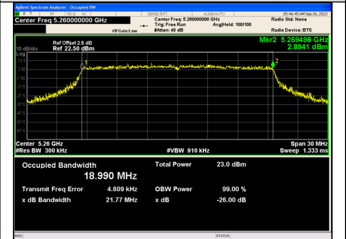
IEEE 802.11ax_Channel 52_20MHz_Antenna 1_RU&Index 242RU61
