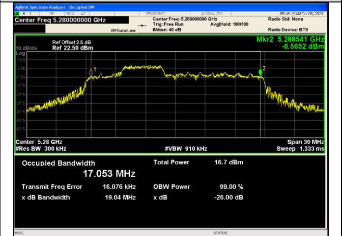
IEEE 802.11ax_Channel 56_20MHz_Antenna 1_RU&Index 52RU38
