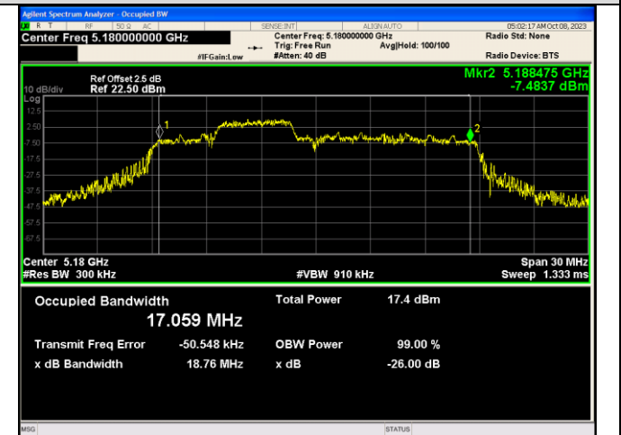
IEEE 802.11ax_Channel 36_20MHz_Antenna 1_RU&Index 52RU38
