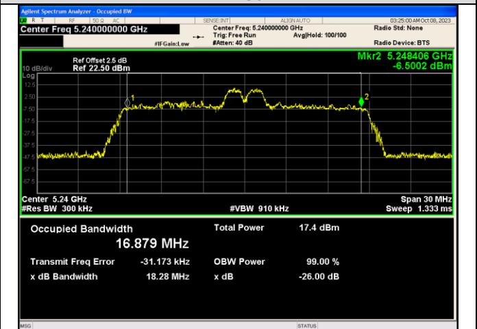
IEEE 802.11ax_Channel 48_20MHz_Antenna 1_RU&Index 26RU4
