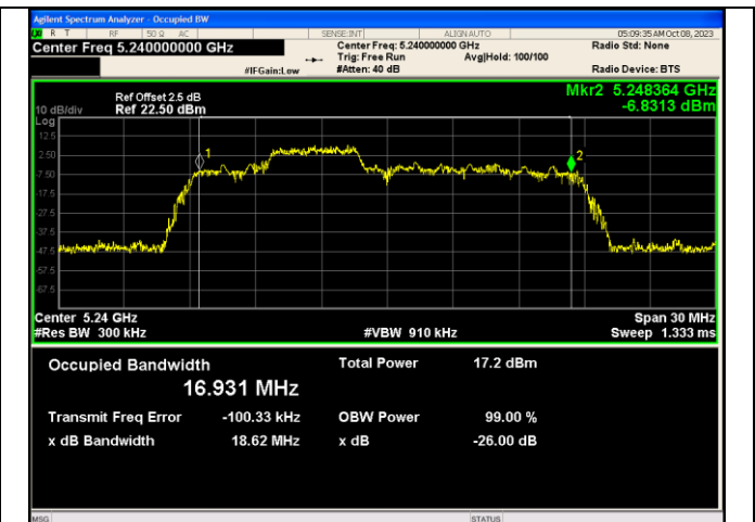
IEEE 802.11ax_Channel 48_20MHz_Antenna 1_RU&Index 52RU38
