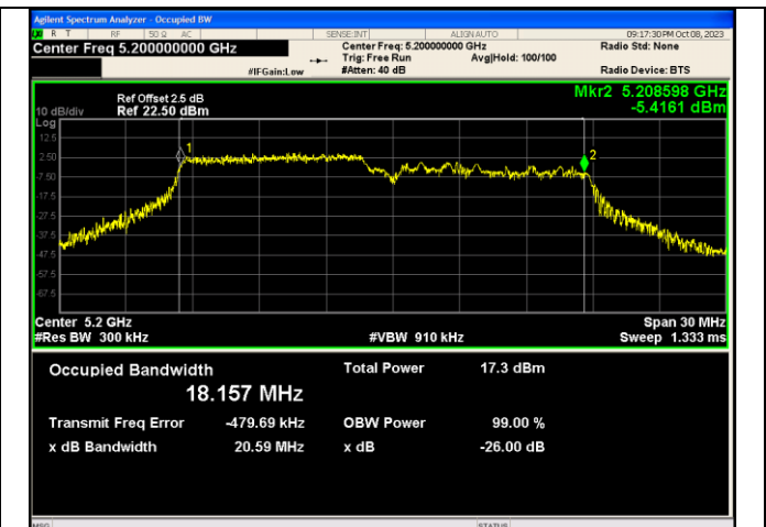
IEEE 802.11ax_Channel 40_20MHz_Antenna 1_RU&Index 106RU53
