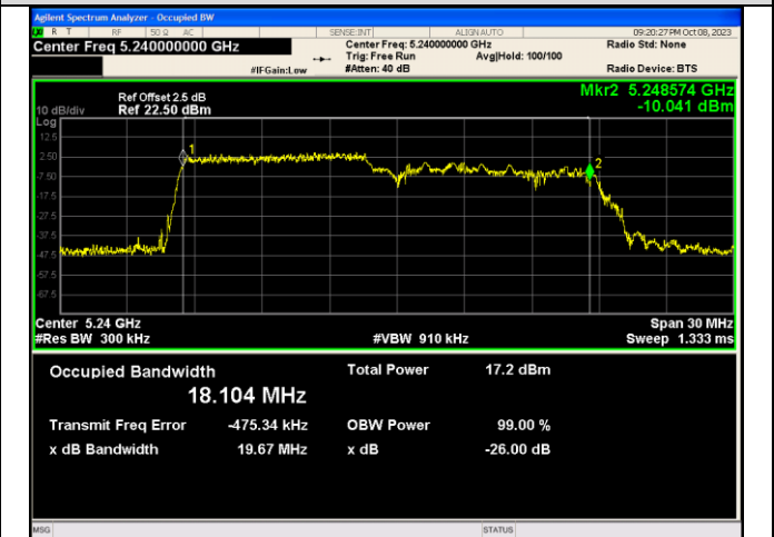
IEEE 802.11ax_Channel 48_20MHz_Antenna 1_RU&Index 106RU53
