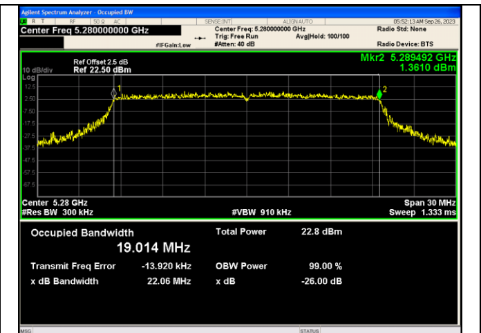
IEEE 802.11ax_Channel 56_20MHz_Antenna 1_RU&Index 242RU61
