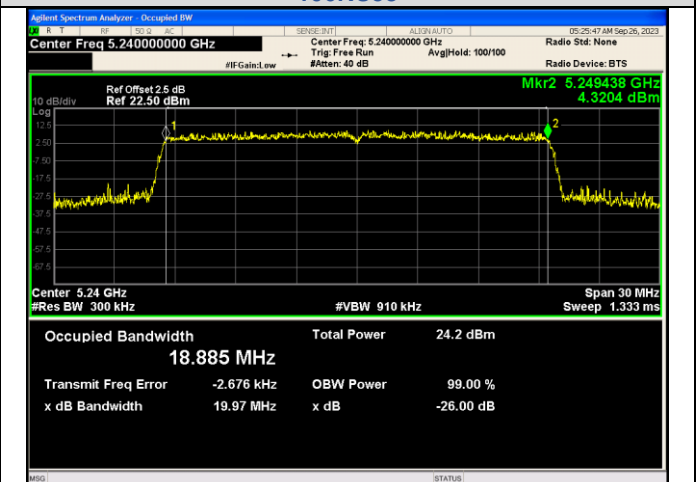
IEEE 802.11ax_Channel 48_20MHz_Antenna 1_RU&Index 242RU61
