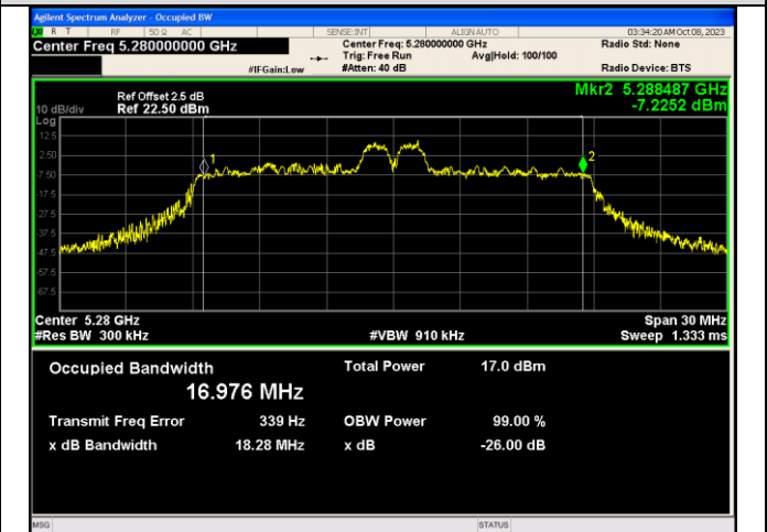
IEEE 802.11ax_Channel 56_20MHz_Antenna 1_RU&Index 26RU4
