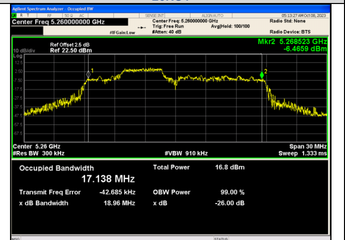
IEEE 802.11ax_Channel 52_20MHz_Antenna 1_RU&Index 52RU38
