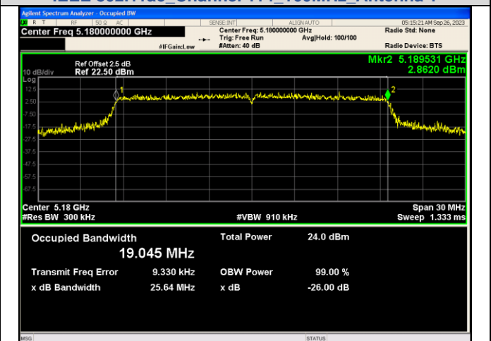
IEEE 802.11ax Channel 36 20MHz Antenna 1_RU&Index 242RU61
