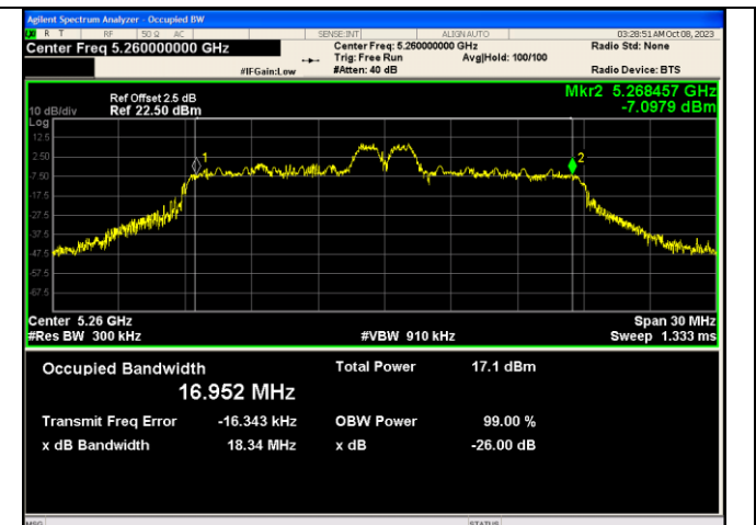
IEEE 802.11ax_Channel 52_20MHz_Antenna 1_RU&Index 26RU4
