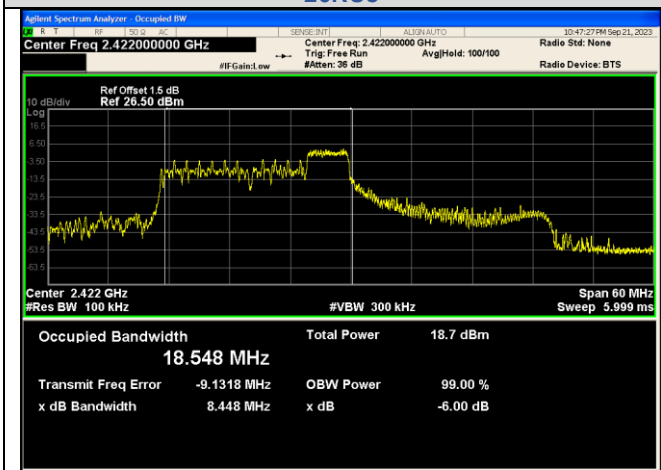
IEEE 802.11ax_Channel 3_40MHz_Antenna 0_RU&Index 52RU40
