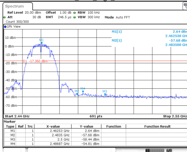
11B_Ant0_High_2462
