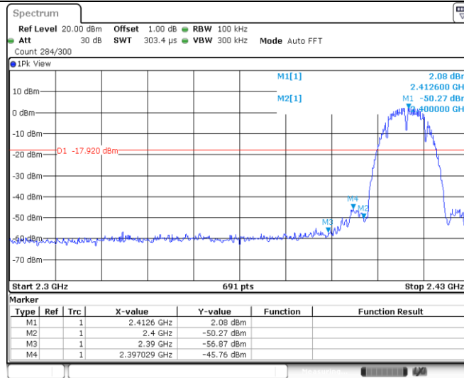
11B_Ant0_Low_2412
