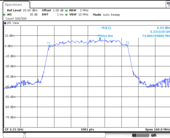
11AC80SISO_Ant1_5210
