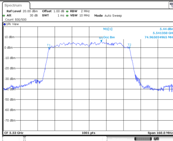
11AC80SISO_Ant1_5530
