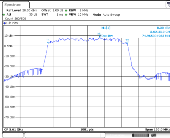
11AC80SISO_Ant1_5610
