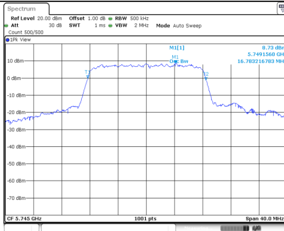
11A_Ant1_5745
