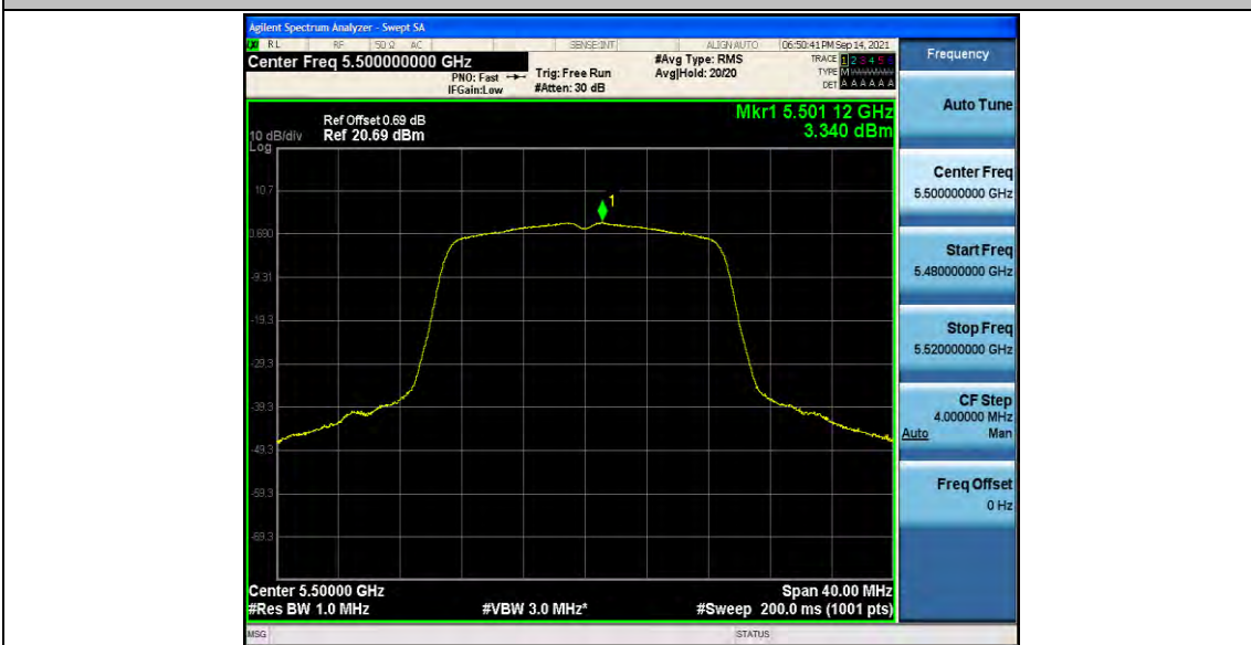
11AC20MIMO_Ant2_5500
