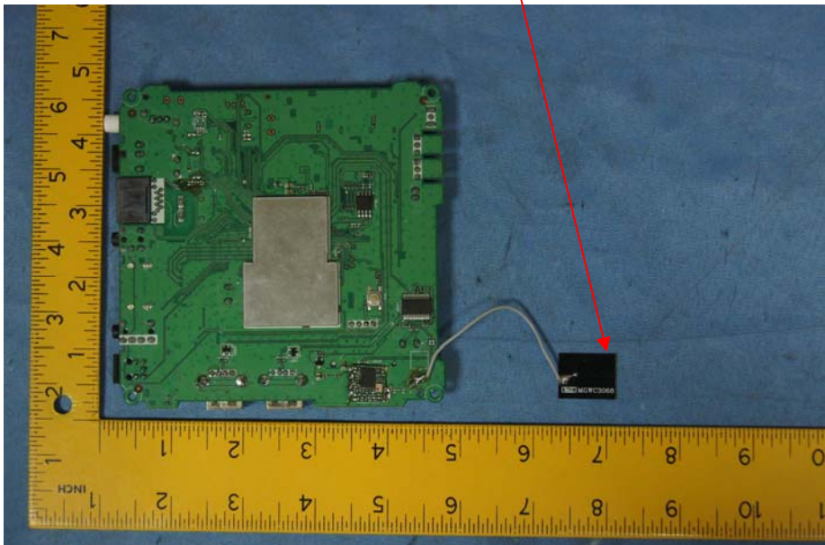
Antenna
