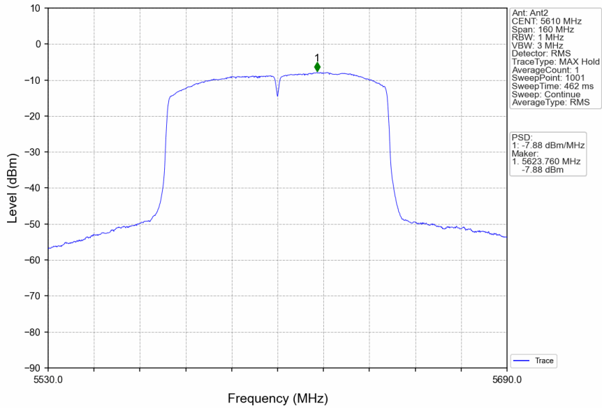
802.11ac(VHT80)_HCH_5610MHz_MIMO_NTNV
