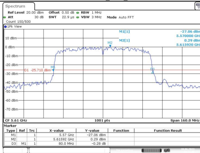
11AC80MIMO_Ant2_5610
