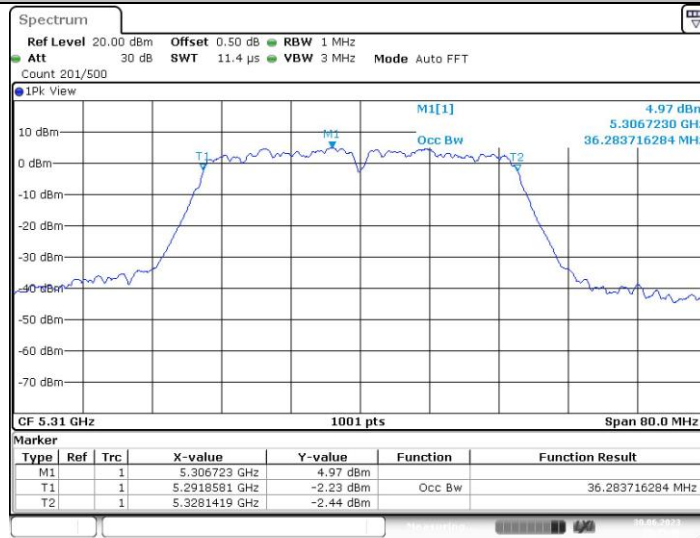
11N40MIMO_Ant2_5310
