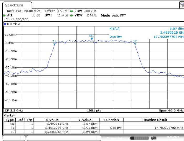
11AC20MIMO_Ant2_5500
