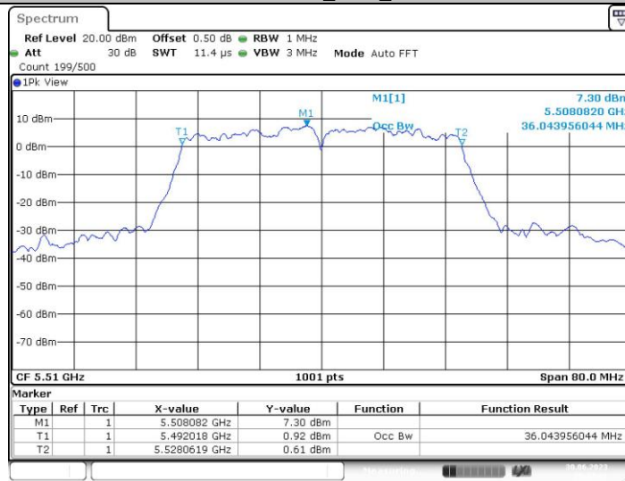
11N40MIMO_Ant1_5510
