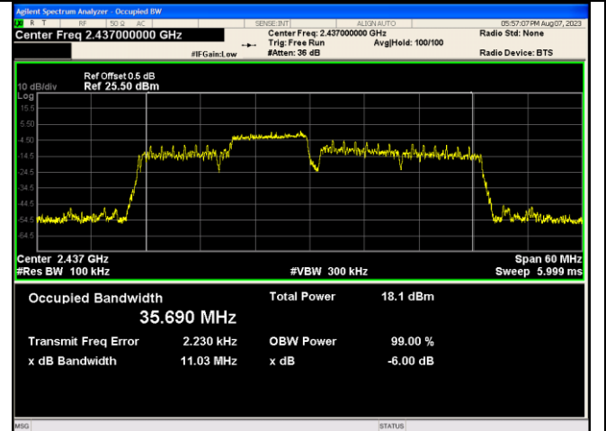
IEEE 802.11ax_Channel 6_40MHz_Antenna 1_RU&Index 106RU54
