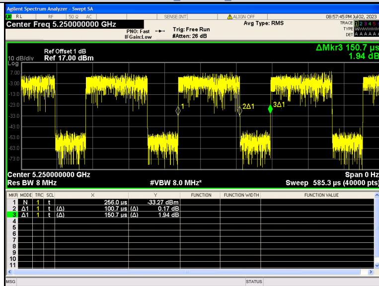
IEEE 802.11ac 160MHz Channel 50
