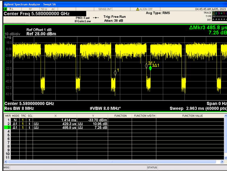
IEEE 802.11ax 20MHz Channel 116
