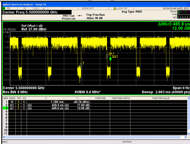
IEEE 802.11ax 20MHz Channel 100
