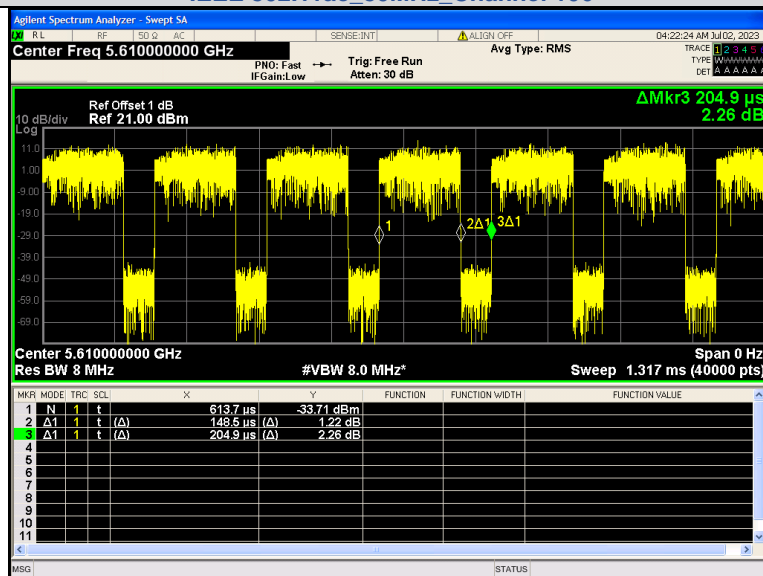
IEEE 802.11ac 80MHz Channel 122
