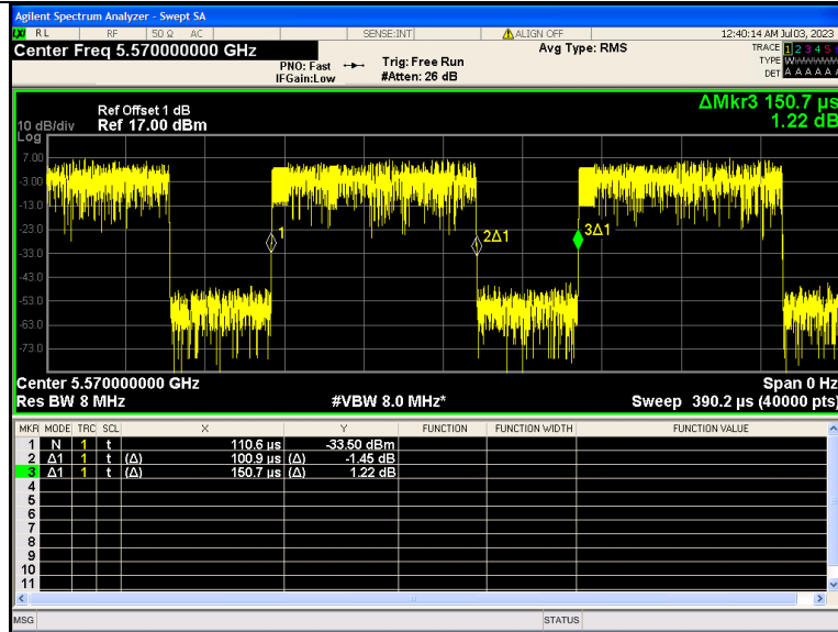
IEEE 802.11ac 160MHz Channel 114
