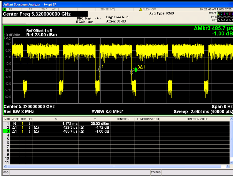
IEEE 802.11ax 20MHz Channel 64
