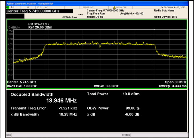
IEEE 802.11ax Channel 149 20MHz Antenna 1 RU&Index 242RU61
