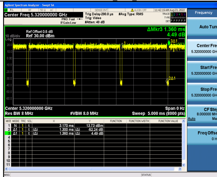
11N20MIMO_Ant2_5320
