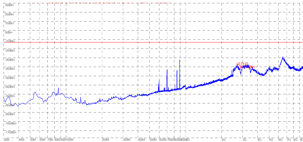
(Plot A: Test Antenna Horizontal)
