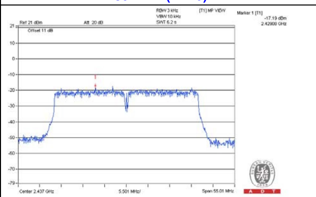
802.11n (HT40)
