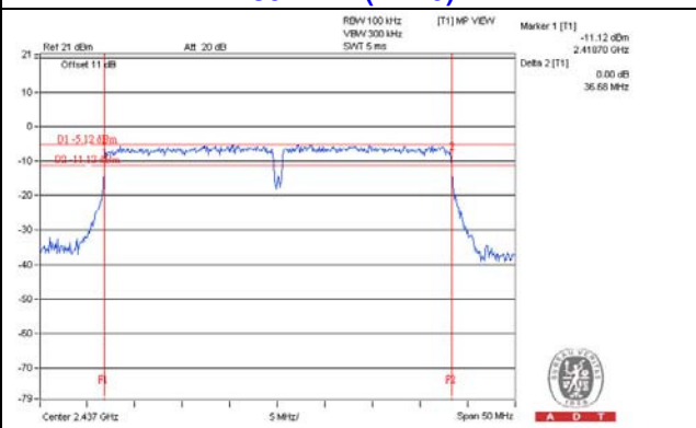
802.11n (HT40)
