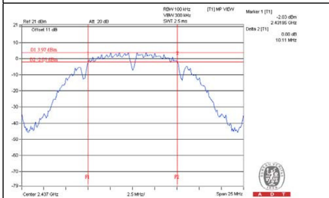
802.11n (HT20)
