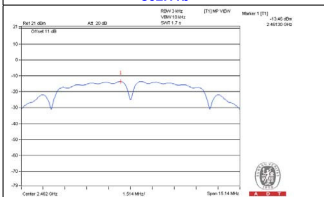
802.11n (HT20)
