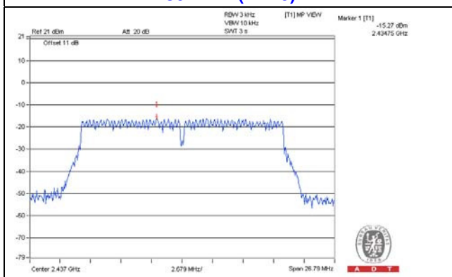
802.11n (HT20)
