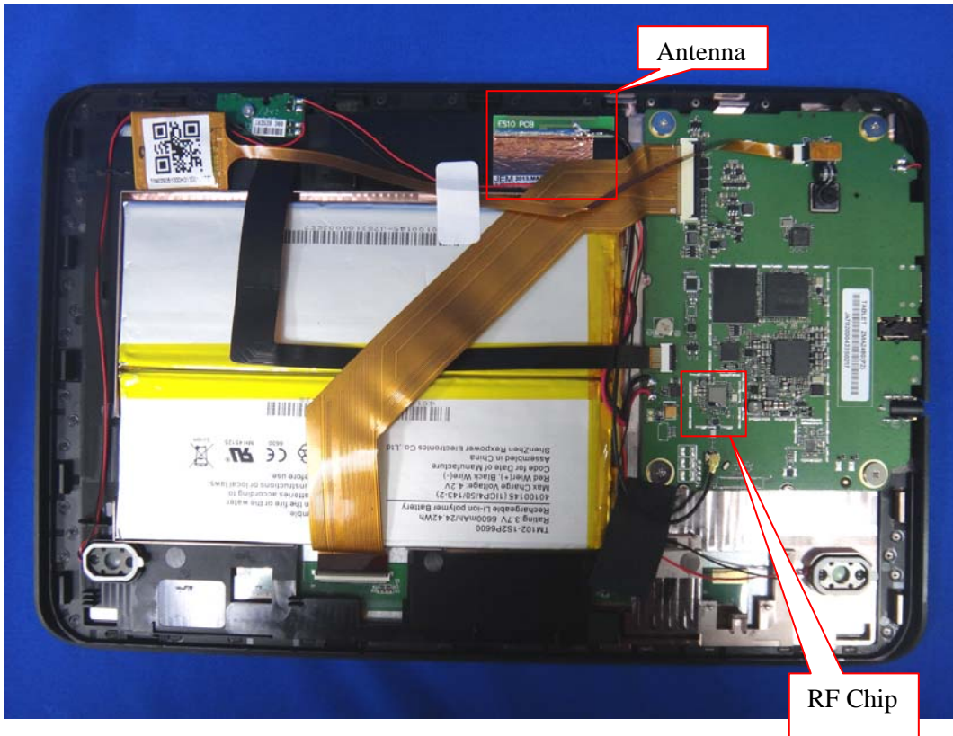
(6) EUT Photo (Antenna)
