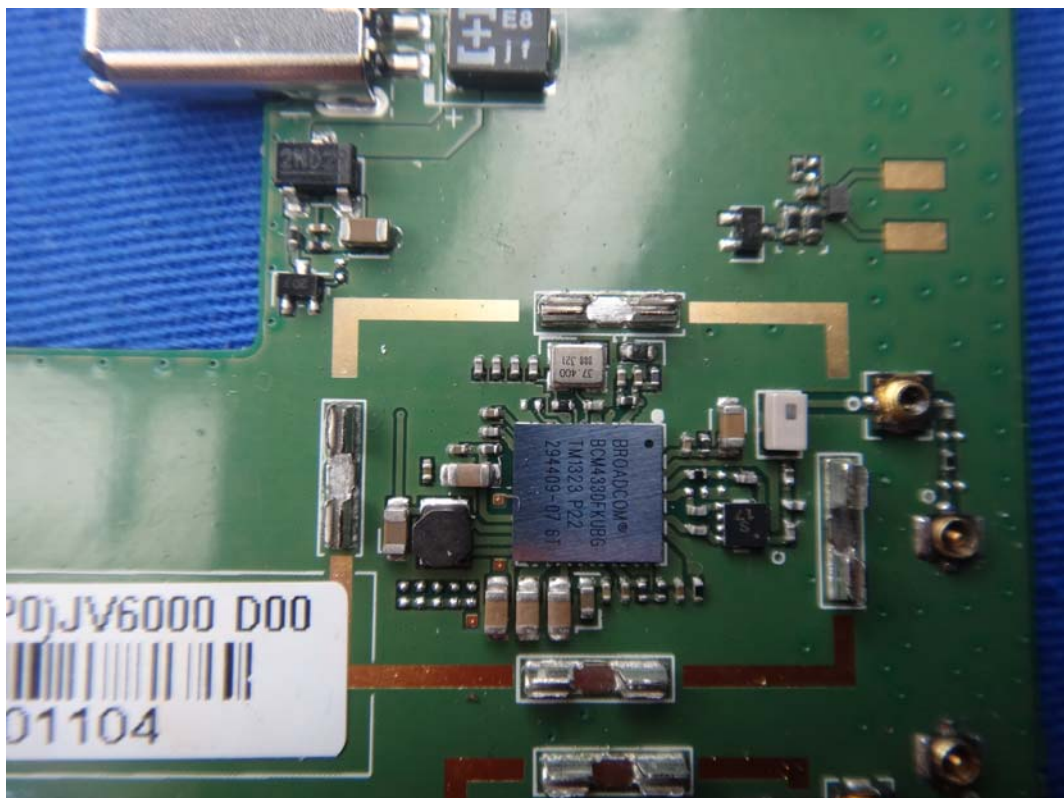
(6) EUT Photo WLAN+Bluetooth IC
