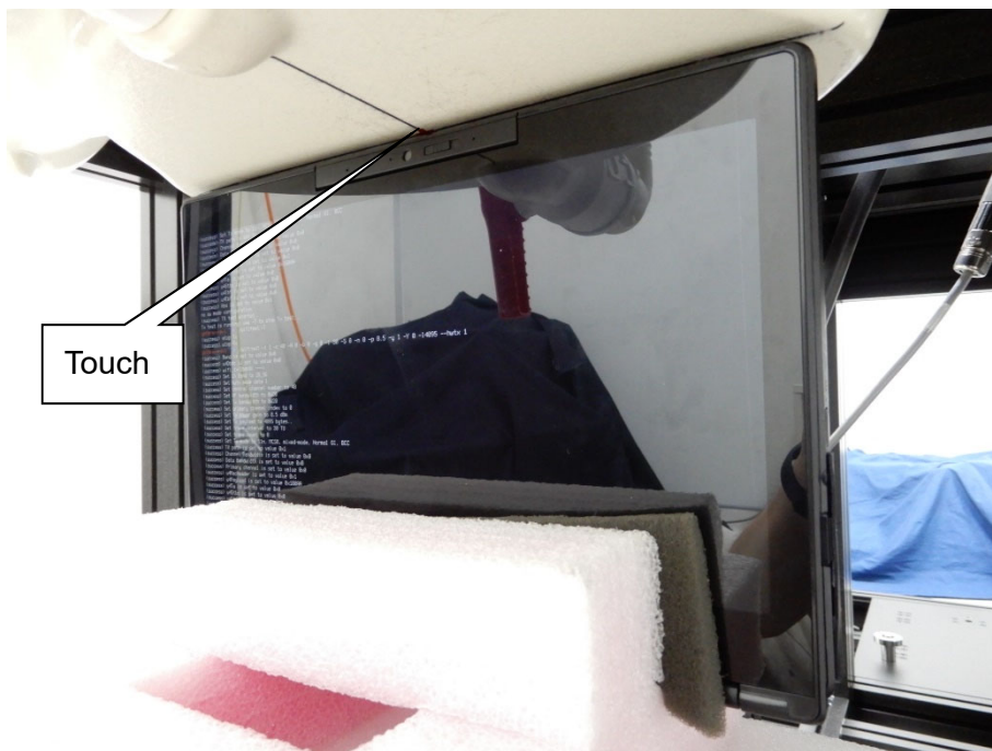
EUT Top(PAD)
