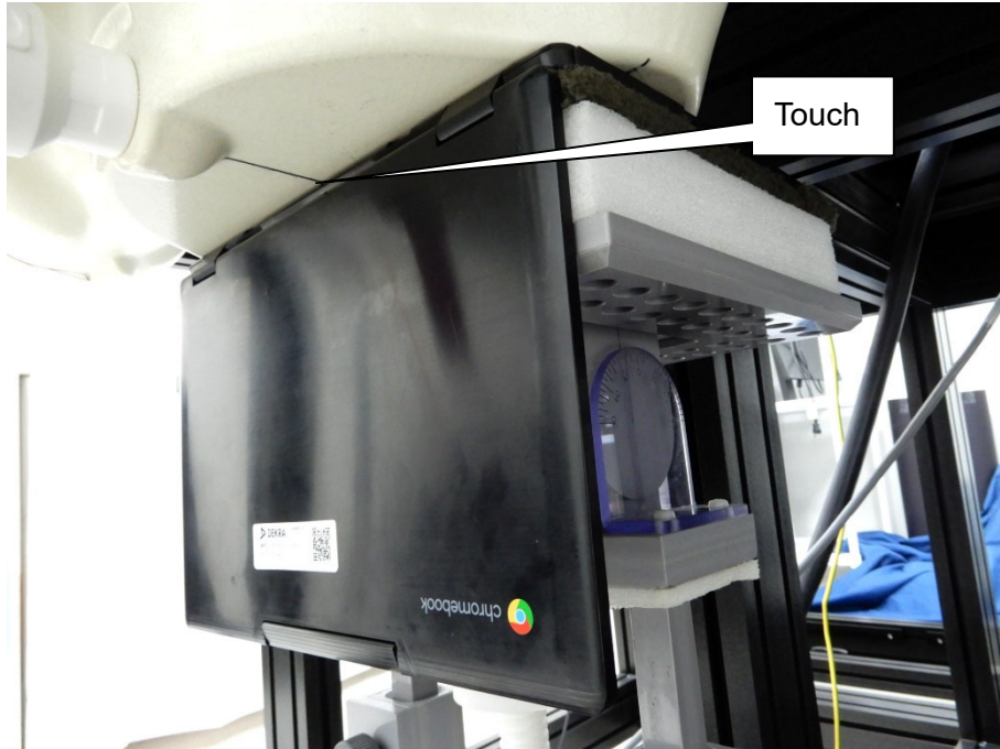
EUT Bottom(NB)
