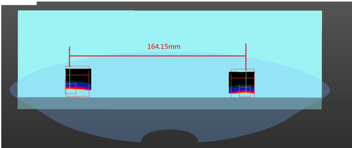
5G(M+A) - Back(PAD)
