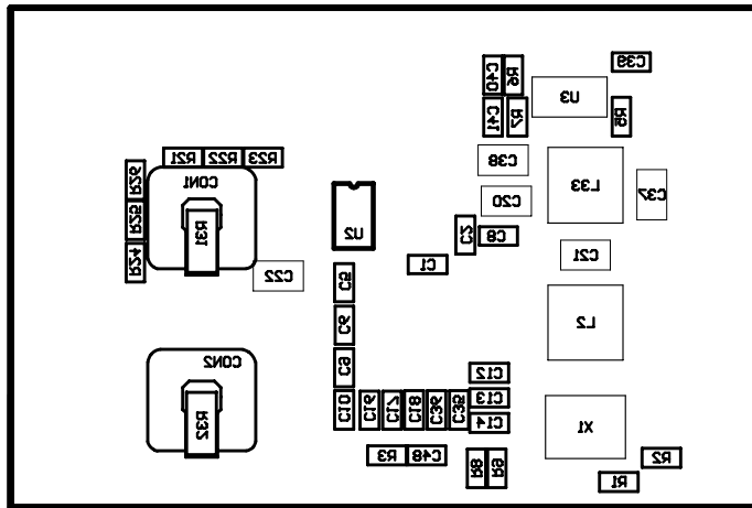
Bottom Overlay
