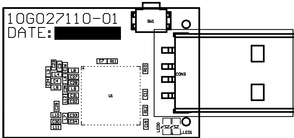
Top Overlay
