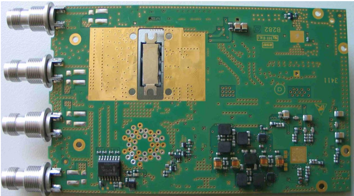
PA Module Bottom
