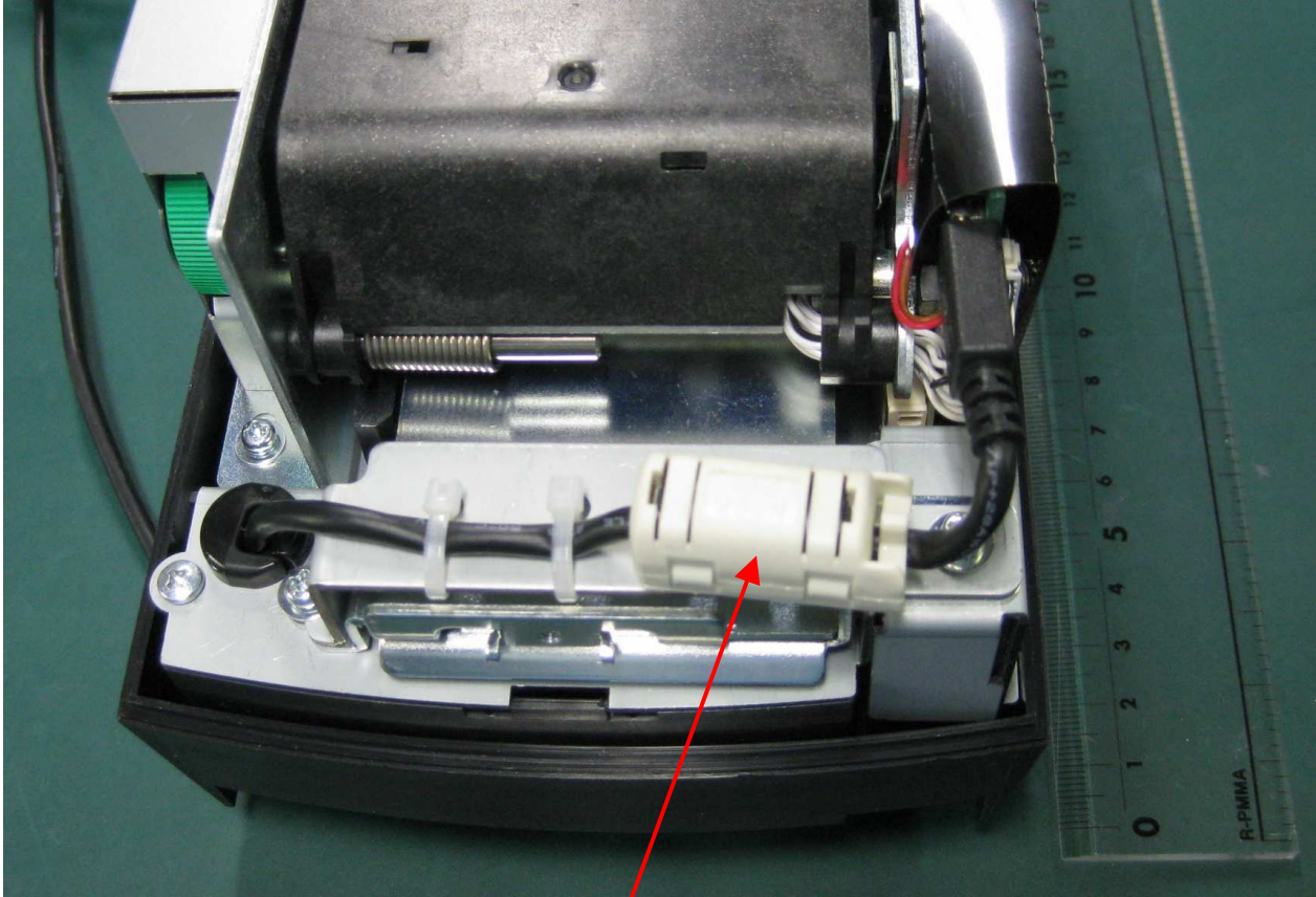
Ferrite core : SFT-25SN(TKK)
