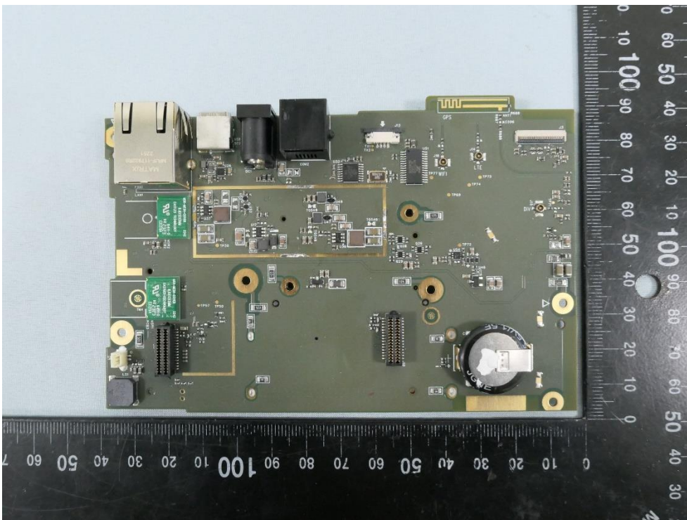
(30) EUT Photo
